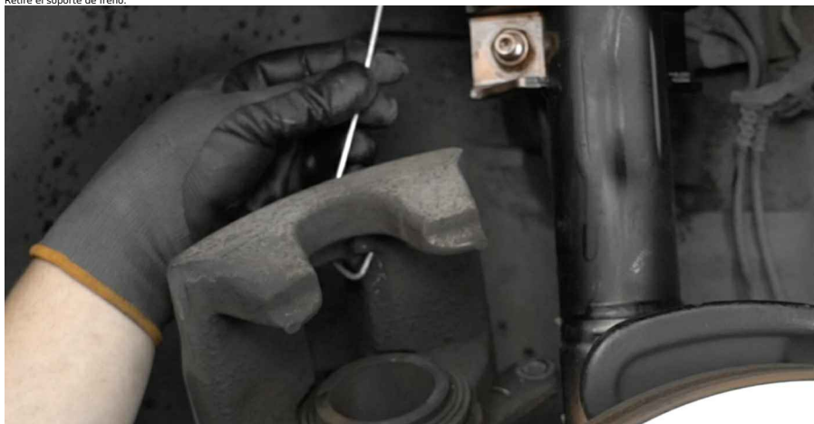
Sustitución: sensor de desgaste de pastillas de frenos - MERCEDES-BENZ Clase E Cabrio (A207). Consejo:
