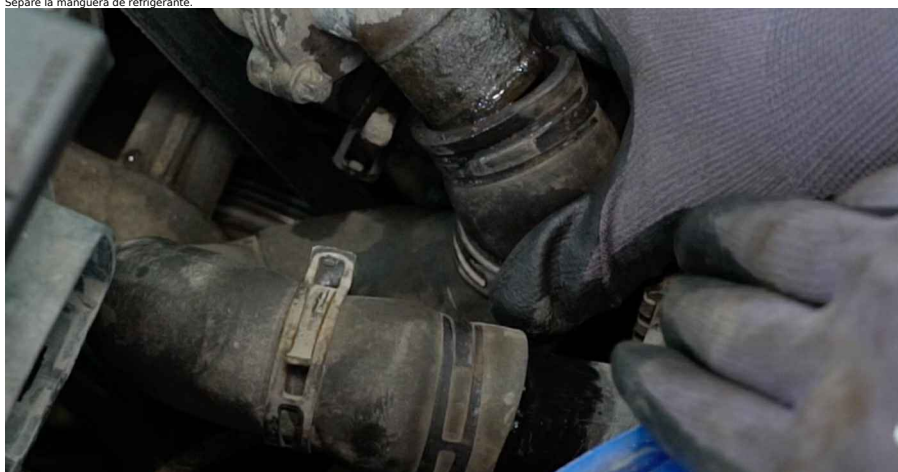
Sustitución: termostato refrigerante - VAUXHALL Astra Mk1 Familiar. AUTODOC recomienda: • ¡Cuidado! El refrigerante podría fugarse de las líneas de refrigerante y de la carcasa del termostato.
