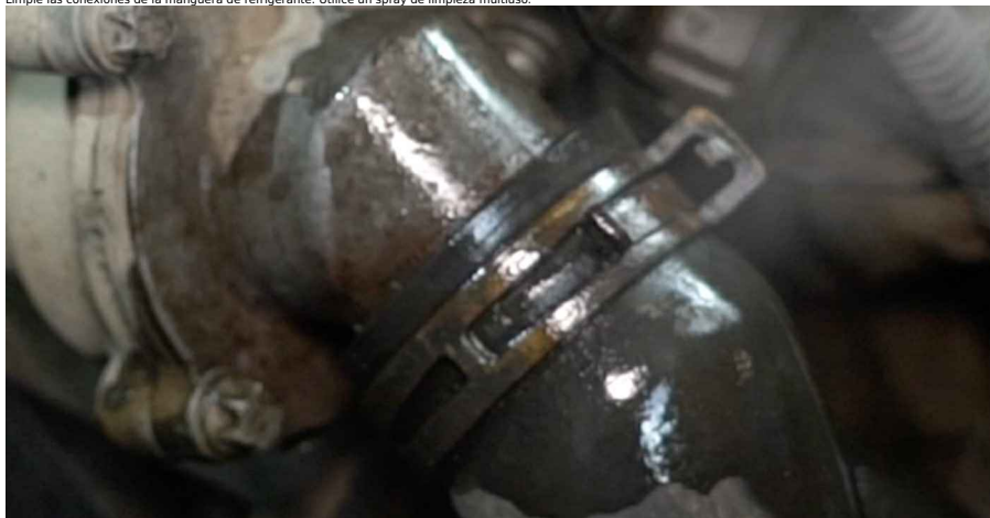
16 Afloje las abrazaderas de las mangueras de refrigerante. Utilice alicates para abrazaderas clic-R.
