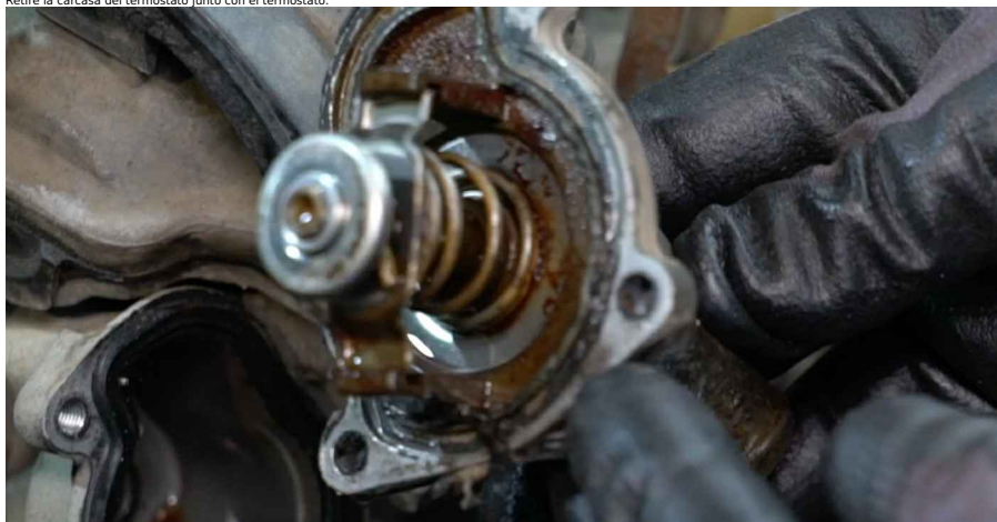
22 Cubra el asiento de montaje de la carcasa del termostato mediante un paño de microfibra para evitar la entrada de suciedad y objetos extraños en el sistema.
