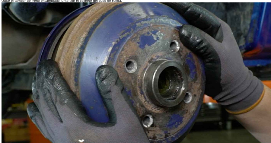
Sustitución: cojinete de rueda - VAUXHALL Cavalier Mk2 Berlina (j82). Consejo de AUTODOC:
