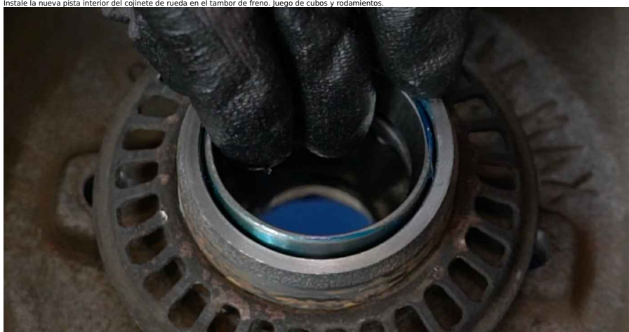
19 Instale la nueva pista interior del cojinete de rueda en el tambor de freno. Juego de cubos y rodamientos.
