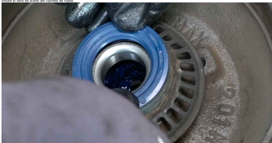
23 Trate el eje de la mangueta. Utilice un spray de limpieza multiuso. Utilice grasa para rodamientos.
